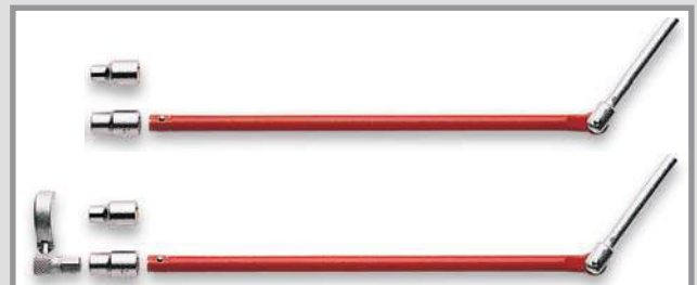
Art.Nr. 013025 Artikelbezeichnung Standhahn-Mutter-Steckschlüssel DBGM mit Steckschlüsseleinsatz 10/13mm, Antrieb 1/2"
